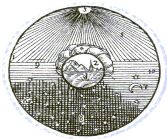
Figura 4. Geocentrismo.
